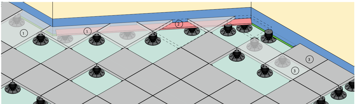
Abb. 8: Anordnung von Stelzlageren unter Anschnittplatten; (1) Anschnittplatten Variante mit grösserem Plattenformat, (2) Metallprofil, (3) Anschluss mit Normalplatten auf 2 oder 3 Plattenreihen verteilt
